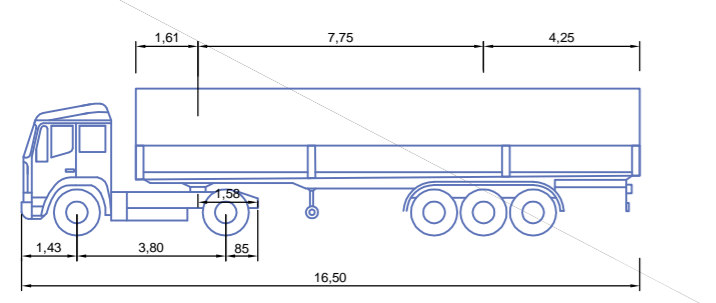
Bemessungsfahrzeug SATTELZUG lg=16,50m
